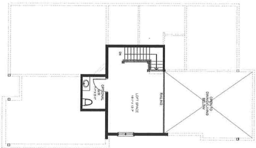
LOFT PLAN
